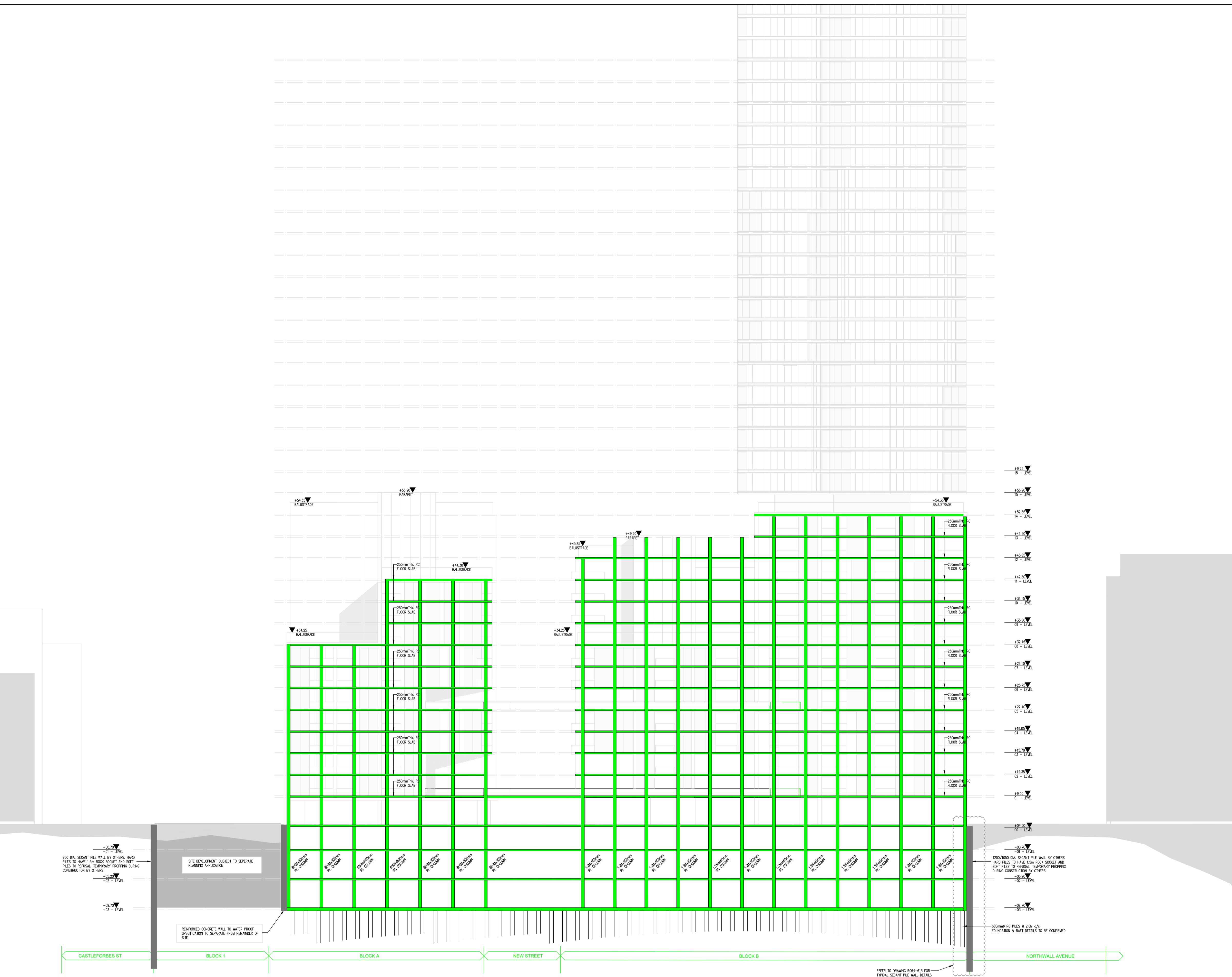
SECTION A-A SCALE: 1/300
